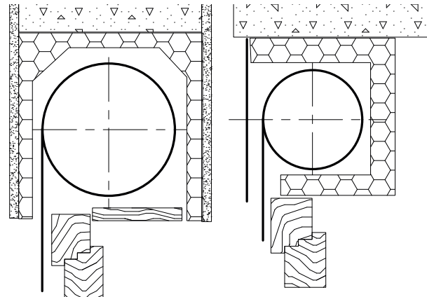
Einbaurollladen
