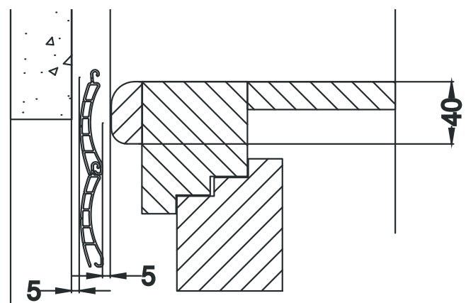
Beispiel für die Gestaltung des Einlaufs, die Abrundung sollte möglichst groß sein. Die Abstandsmaße (5 mm) zur Nennstärke der Rollroststäbe sind wärmetechnisch bedingt (siehe TR 103 Kästen)
